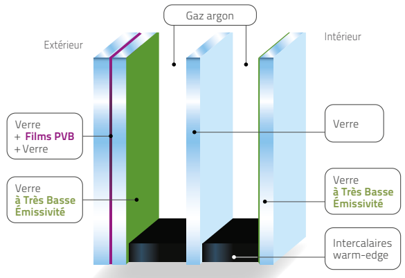
Triple vitrage sécurité : Frappe 44.6 TBE/18/4/18/TBE 4
